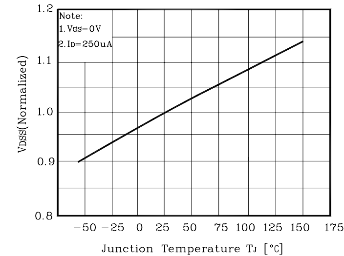
Fig. 7 V_{DS} - T_J
